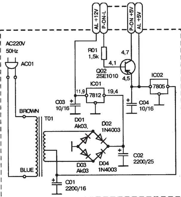
Принципиальная схема источника питания видеоплеера VIP-3000HC/5000HC
